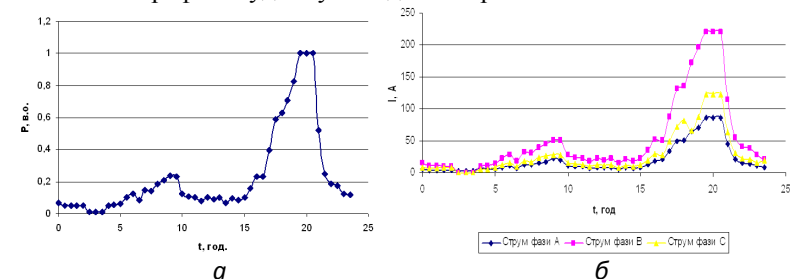
Рис. 1 – Типові графіки 9-ти поверхового будинку: а - навантаження; б - струм
