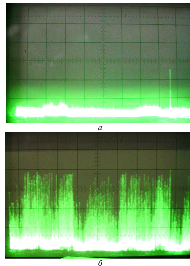
Рис.3 – Фото осциллограммы шумов схемы: a – до начала работы б – после. Цена делений: по горизонтали 2 мс/дел; по вертикали 1 В/дел, что соответствует 1 пКл/дел (При общем усилении 77 дБ: 20 дБ (предварительный усилитель) + 80 дБ (основной усилитель) – (1+2+4+16) дБ (ослабление) = 77 дБ.
