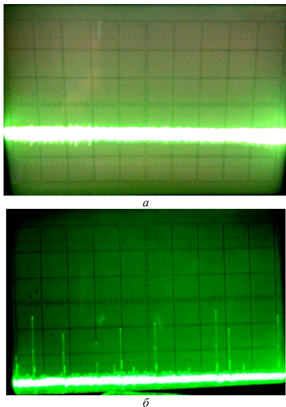
Рис.2 – Фото осциллограммы шумов схемы: a – отключенном основном оборудовании и осветительных люминесцентных ламп типа ДРЛ; б – при включенных лампах типа ДРЛ. Цена делений: по горизонтали 2 мс/дел; по вертикали 2 В/дел, что соответствует 2 пКл/дел (При общем усилении 89 дБ: 20 дБ (предварительный усилитель) + 100 дБ (основной усилитель) – (1+2+4+16+8) дБ (ослабление) = 89 дБ.
