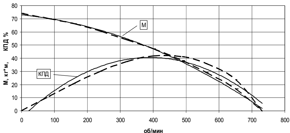
Рис. 2 – Енергетическая характеристика турбобура ТВМ-195 диаметром 195 мм: ---- расчет, - - - эксперимент
