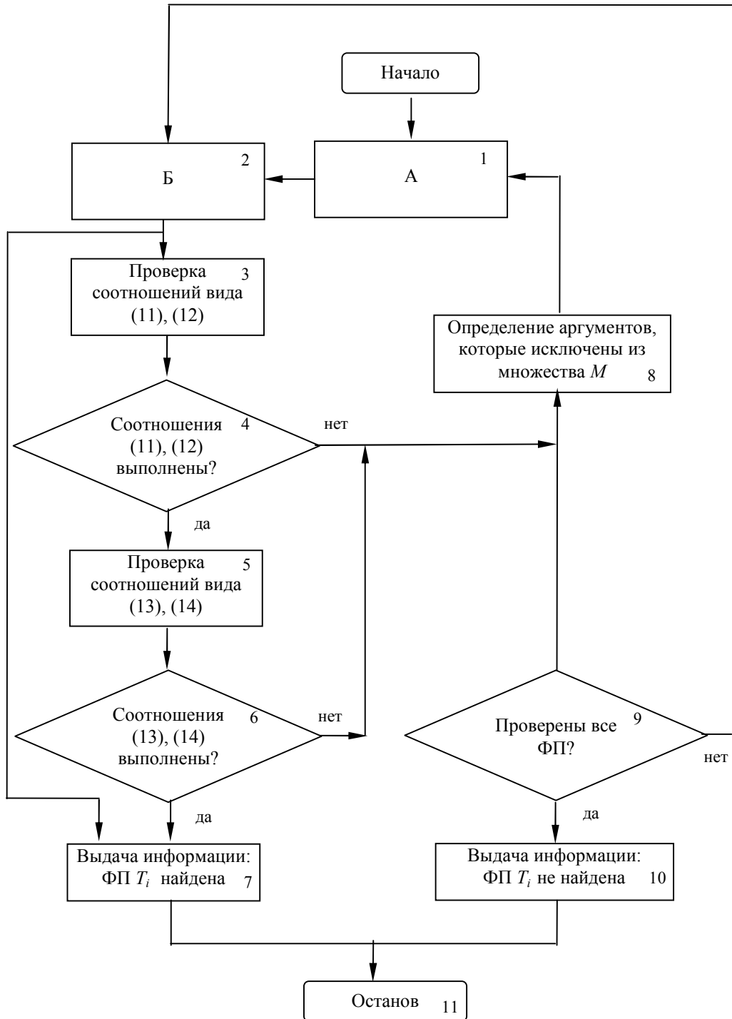
Рис. Обобщенный многоядный алгоритм МГУА для поиска ФП
