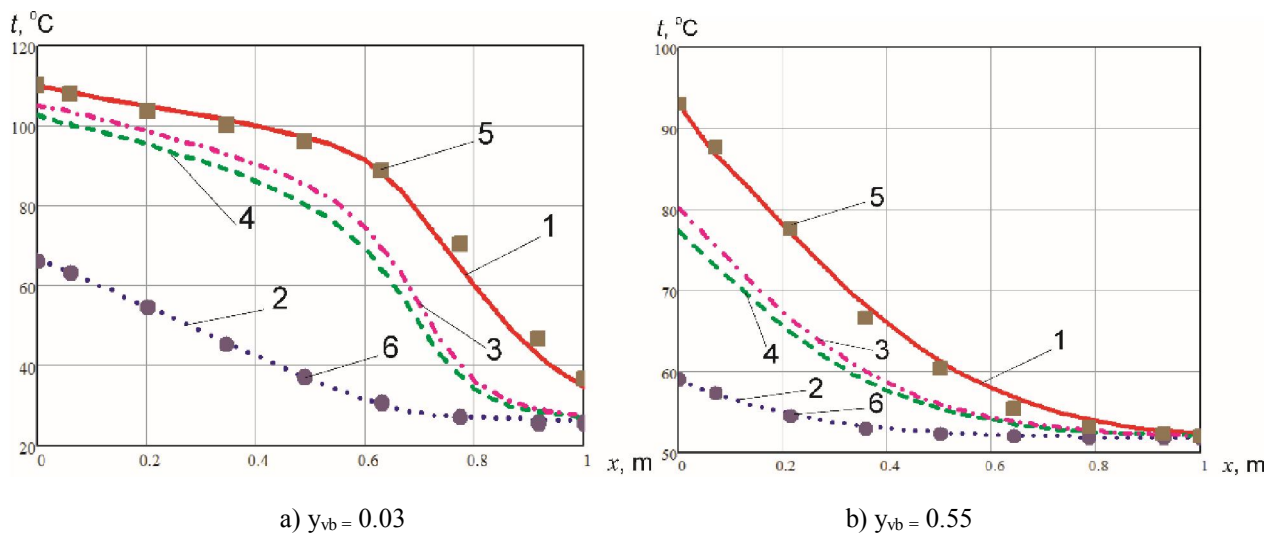
Рисунок 1 – Распределение температур в канале ПТО. Расчетные кривые: 1 – воздушно-паровая смесь; 2 – охлаждающая вода; 3 – пленка конденсата; 4 – стенка. Экспериментальные точки: 5 – воздушно-паровая смесь; 6 – охлаждающая вода.
