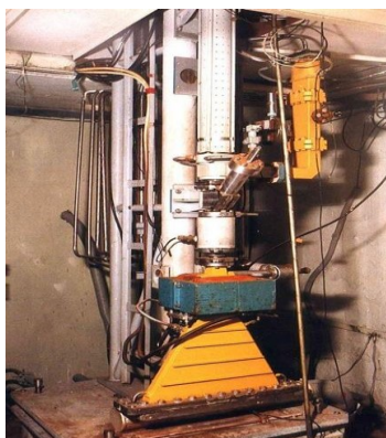
Рис. 3 – Лінійний прискорювач електронів КУТ–1 на енергію до 10 МеВ (ННЦ “ХФТІ”, 1993 р.) [9].
