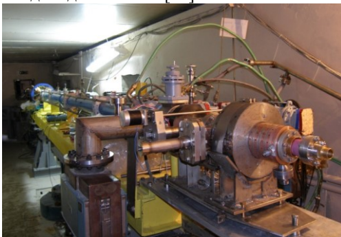
Рис. 4 – Лінійний прискорювач електронів ЛПЕ-60-М на енергію до 100 MeV (ННЦ “ХФГГ”, 2008 р.) [9].
