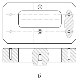
Рисунок 3 – Опорную часть рамы в месте установки колес: а – с ребрами чугунной рамы болтовыми соединениями; б – вставки из стали 09Г2С
