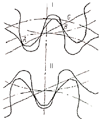
Рисунок 1 – Початок зачеплення (I) та положення мінімального замкненого об'єму (II) при зачепленні без зазорів
