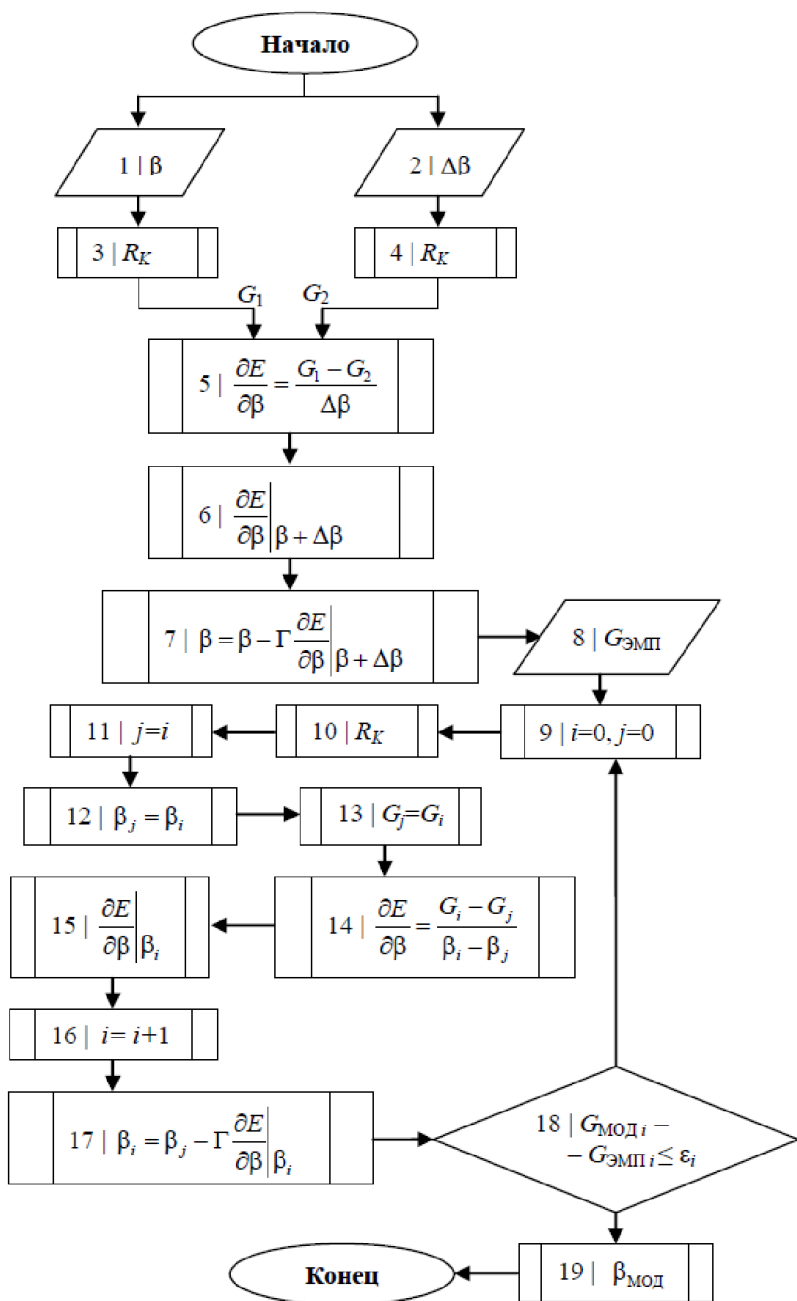
Рисунок – Блок-схема алгоритма настройки параметров модели.
