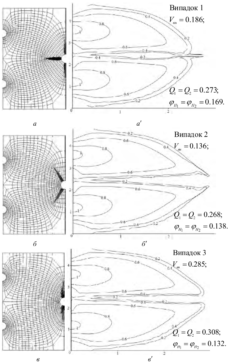
Рис. 2 – Гідродинамічні сітки ( a , б , в ) та, відповідні їм, розподіли насиченості елементів симетрій у момент часу \tilde{t} = 4.64 ( a' ), \tilde{t} = 4.92 ( б' ), \tilde{t} = 5.98 ( в' ).
