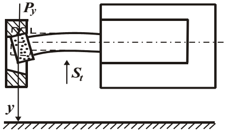
Рис. 1 – Розрахункова схема параметрів внутрішнього шліфування.
