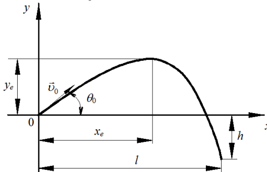
Рис. 1 – Расчётная схема.
