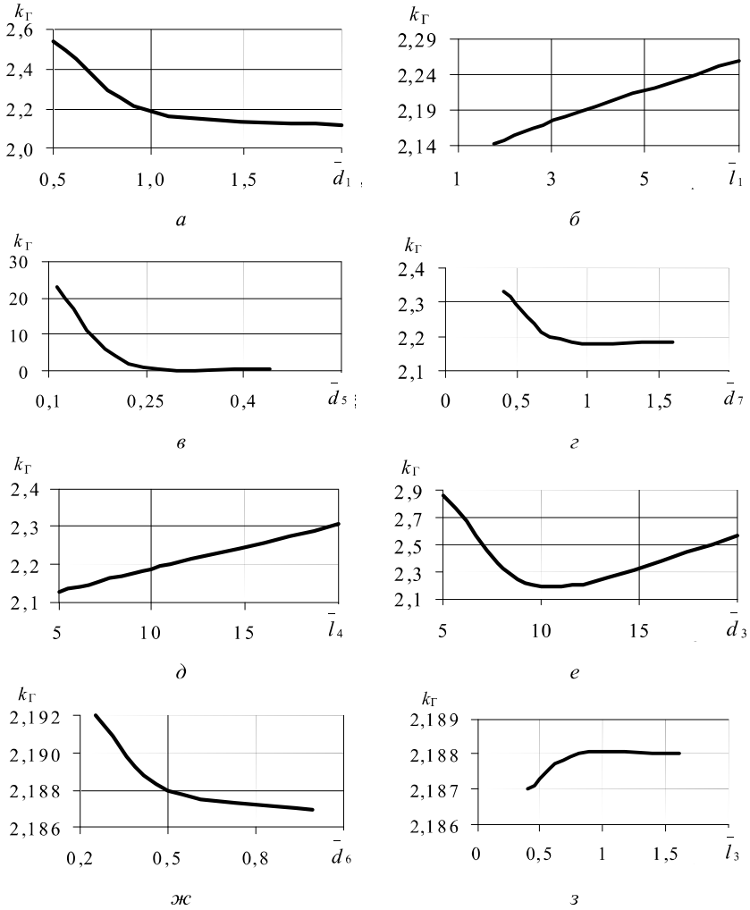
Рис. 2 – Залежність коефіцієнта гасіння ГПТ від відносних конструктивних параметрів: а – діаметра вхідного патрубку \bar{d}_1 ; б – довжини вхідного патрубку \bar{l}_1 ; в – діаметра отвору 5; г – діаметра отвору 7 \bar{d}_5 ; д – половини довжини проточних камер гасителя \bar{l}_4 ; е – внутрішнього діаметра корпусу \bar{d}_3 ; ж – діаметра короткого внутрішнього патрубку \bar{d}_6 ; з – довжини короткого внутрішнього патрубку \bar{l}_3 .
