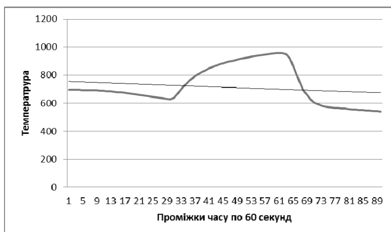
Рис. 6 – експоненціальне усереднення температури у точці Дно 2 на протязі роботи пальників із циклом переключення 30 хвилин
