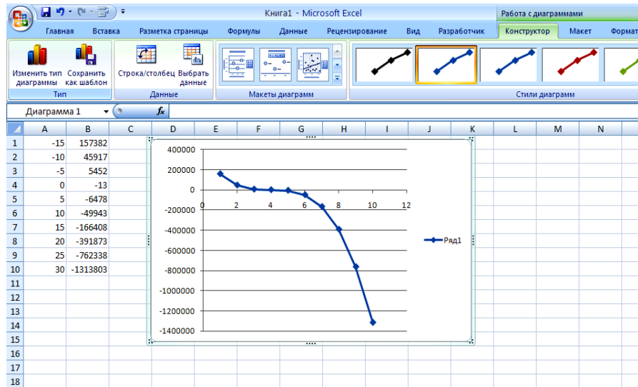
Рис. 3 - Численные значения аргумента x и функции y(x) = -48 \cdot x^3 - 20 \cdot x^2 + 7 \cdot x - 13 на заданном диапазоне и построенный точечный график, выполненный макросом
