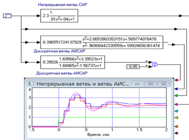
Рис. 2 – Дослідження еквівалентності безперервного і дискретного ланок САР
