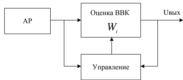
Рис. 4 – Структурная схема оптимального приема i -го сигнала АС
