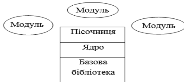
Рис. 1 - Компоненти SPA-застосунку
