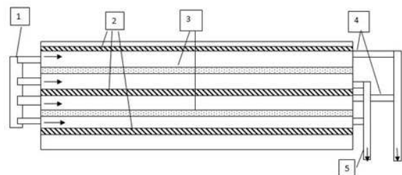
Рис. 5 - Схема проточного активатора воды
