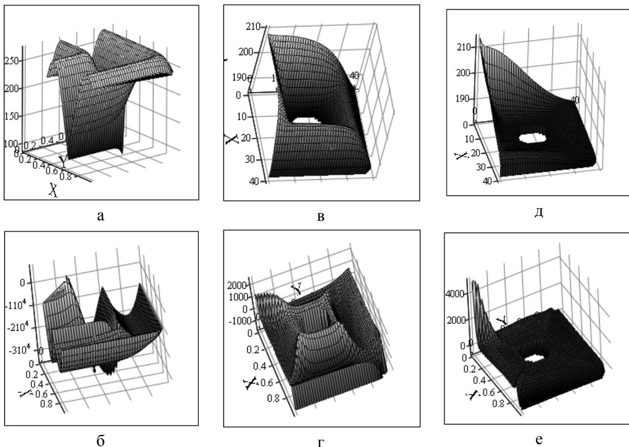
Рис.4 - Температура ПСЭЖ - а, в, д, и правая часть - б, г, е для точного решения (7) ПСЭЖ рис. 1а (а и б), и для точных решений (4) - в, г, и (5) (д, е) для ПСЭЖ рис. 1б.
