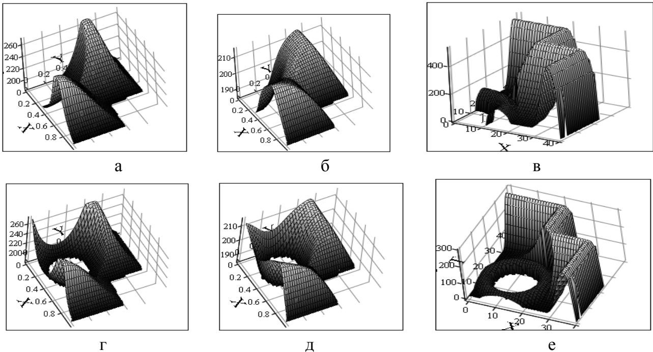
Рис. 6 - Температура ПСЭК рис. 5а (а, б, в) и ПСЭК рис. 5б (г, д, е) для точных решений (1) – (а), (г), (2) – (б), (д) и (7) – (в), (е)
