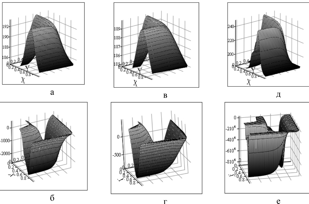
Рис.2 - Температура ПСЭЖ (а, в, д) и правая часть (б, г, е) для точных решений (а), (б) – (1); (в) (г) – (2), (д), (е) – (3)
