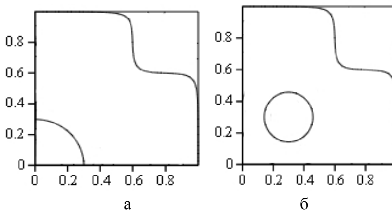
Рис. 5 - ПСЭЖ в виде креста, образованного полосами 1x0.6 с круглым отверстием радиусом 0.3, центр отверстия [0;0] - а и [0.45;0.45] - б
