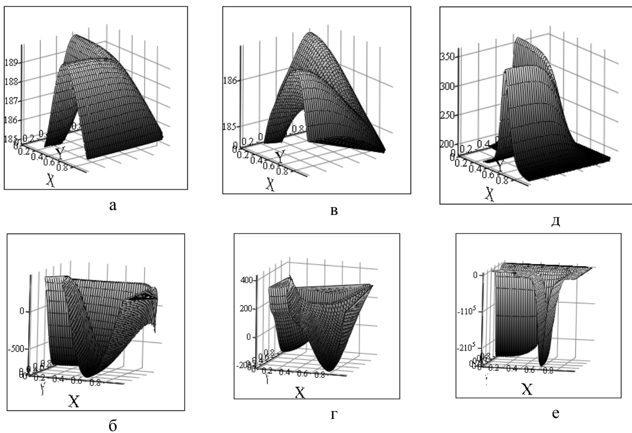
Рис.3 - Температура ПСЭЖ рис. 1а (а, в, д) и правая часть (б, г, е) для точных решений (а), (б) – (4); (в) (г) – (5), (д), (е) – (6)
