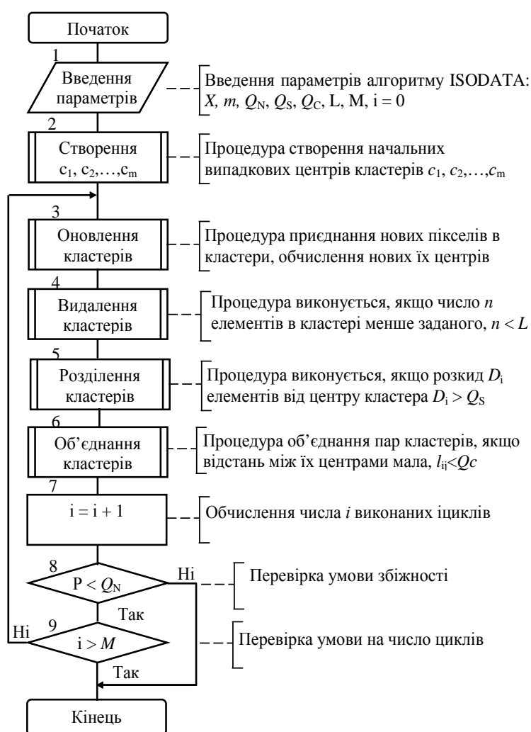
Рис. 1 – Укрупнена схема алгоритму ISODATA
