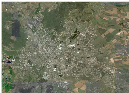
Рис. 2 – Супутниковий знімок території м. Харкова (супутник Landsat 7, дата зйомки: червень 2012, роздільна здатність 30 метрів)
