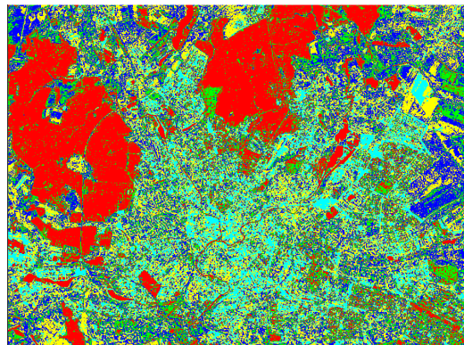
Рис. 3 – Фрагмент знімка території м. Харкова після класифікації
