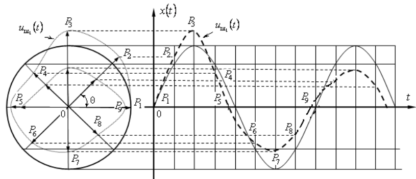
Рис. 1 - Процесс формирования хаотического сигнала x_{\text{xc}}(t) на основе синусоидального колебания
