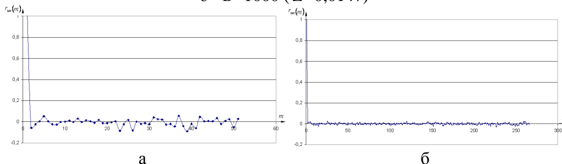
Рис. 4 - Нормированная АКФ шумового сигнала на основе изменения амплитуды U_{ш}(t) по экспоненциальному закону распределения для значений: а - B=100 ( Z=0,0541 ); б - B=1000 ( Z=0,0369 )
