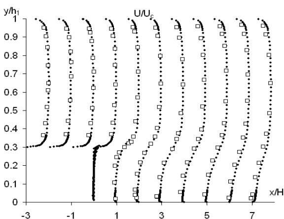
Рис. 2 - Распределение по высоте продольной скорости для канала без преграды; \bullet\bullet\bullet – расчет, \square\square\square – эксперимент
