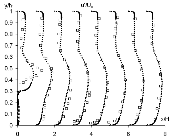
Рис. 5 - Распределение по высоте среднеквадратичной пульсации скорости для канала с преградой; \bullet\bullet\bullet – расчет, \square\square\square – эксперимент
