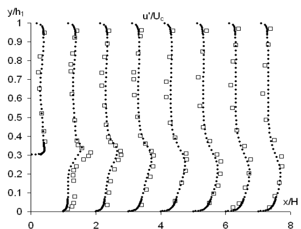
Рис. 3 - Распределение по высоте среднеквадратичной пульсации скорости для канала без преграды; \bullet\bullet\bullet – расчет, \square\square\square – эксперимент
