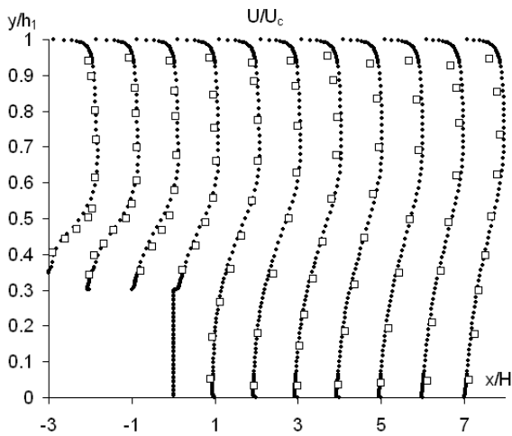
Рис. 4 - Распределение по высоте продольной скорости для канала с преградой; \bullet\bullet\bullet – расчет, \square\square\square – эксперимент
