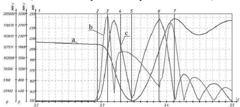
Рис. 4 - График линейного перемещения скорости и ускорения движения штока амортизатора: a – перемещение; b – скорость; c – ускорение
