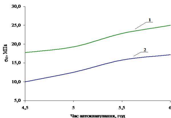
Рис. 1. – Залежність межі міцності при стиску від тривалості ізотермічної витримки 1 – з домішкою склобою; 2 – без домішки
