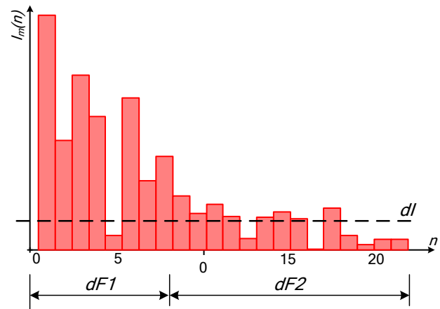
Рис. 2 – До пояснення методики синтезу гібридного накопичувача
