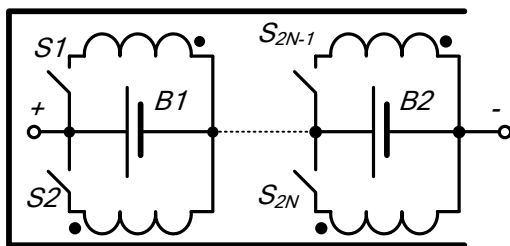
Рис. 7 – Схема активного балансира з адресною передачею заряду (для N акумуляторів)
