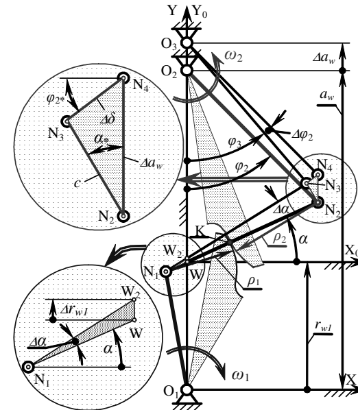
Рисунок 3 – Расчетная схема
