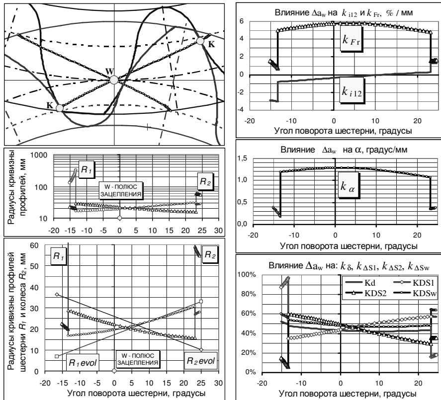
Рисунок 5 – Модифицированная передача с \sigma_H = 1000/750 МПа, a_w = 100 мм, b_2 = 23,44 мм, P = 100 кВт, n_1 = 4000 об/мин: R кривизны профилей; влияние \Delta a_w на работу передачи
