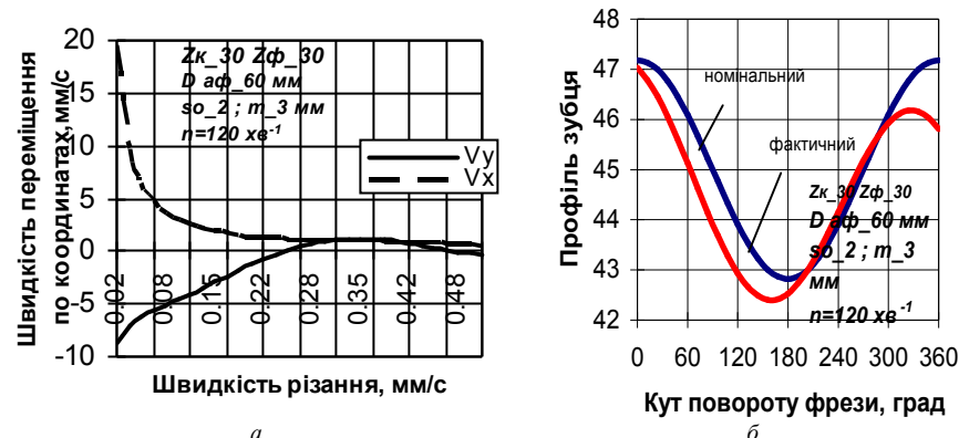
Рисунок 7 – Номінальний та фактичний профіль зубця внаслідок нерівномірності швидкості різання
