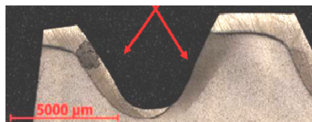
Рисунок 9 – Одностороннее закаленное зубчатое зацепление: фото компании МАТЕХ РМ
