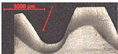
Рисунок 8 – Закаленное зубчатое зацепление с непостоянной толщиной: фото компании МАТЕХ РМ
