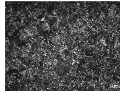
Рисунок 7 – Сталь 12 051, мелкозернистая структура после заковки лазером, Нитал 3%
