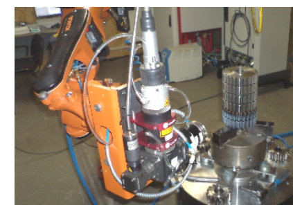
Рисунок 5 – Настройка манипулятора лазера для заковки следующего слоя
