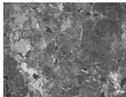
Рисунок 6 – Сталь 12 051, основная структура, Нитал 3%
