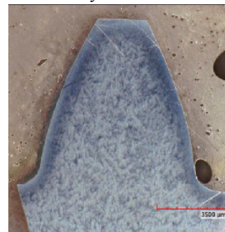
Рисунок 1 – Прокалка зубчатого зацепления
