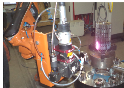
Рисунок 4 – Постепенная заковка зацепления лазерным лучом шириной 40мм
