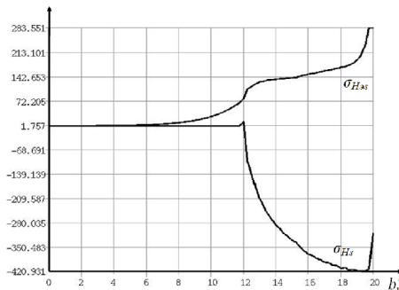
Рисунок 5 – Полученные при моделировании компьютерные графики при \psi = 0,10, \rho_\beta = 338,6, S^* = 9,75
