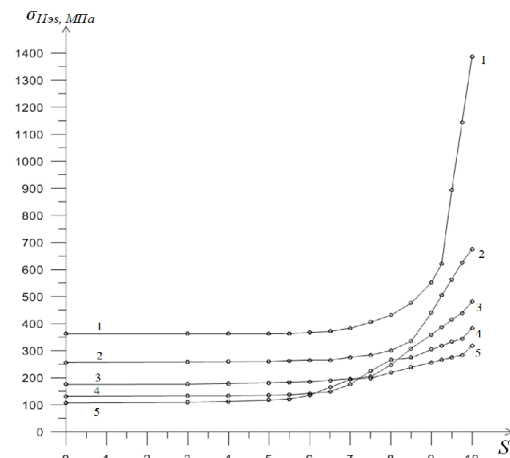
Рисунок 6 – Графики функций фазового эффективного напряжения \sigma_{H\beta} = f(S^*) : 1 – \psi = 0,05 ; 2 – \psi = 0,1 ; 3 – \psi = 0,15 ; 4 – \psi = 0,2 ; 5 – \psi = 0,25
