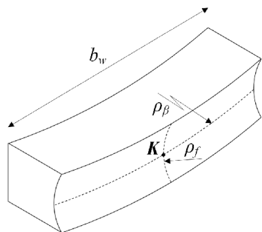
Рисунок 1 – Общий вид упругого индентора, K – одна из теоретических точек контакта гиперболического типа
