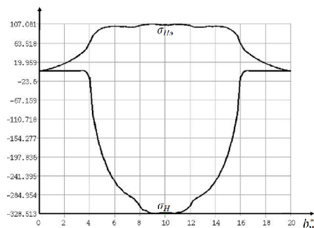
Рисунок 3 – Полученные при моделировании компьютерные графики при \psi = 0,25, \rho_\beta = 3784, S = 0
