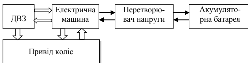
Рис. 2 – Структурна схема гібридної установки з електричною машиною потужністю до 25 кВт
