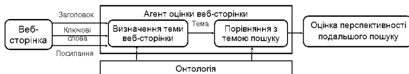
Рис.4 – Оцінювання веб-сторінки на основі методу компараторної ідентифікації
