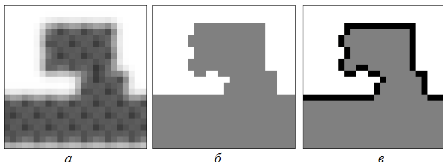
Рис. 3 – Этапы работы алгоритма обнаружения поверхности для сложных поверхностей: а – срез карты электронной плотности, б – срез массива характеристик до нахождения поверхности, в – обработанный массив характеристик
