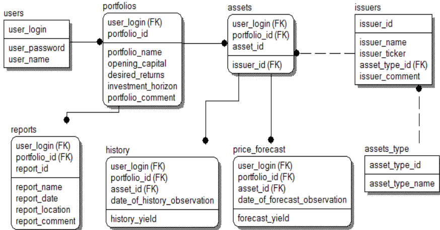
Рис. 3 – Модель даних
