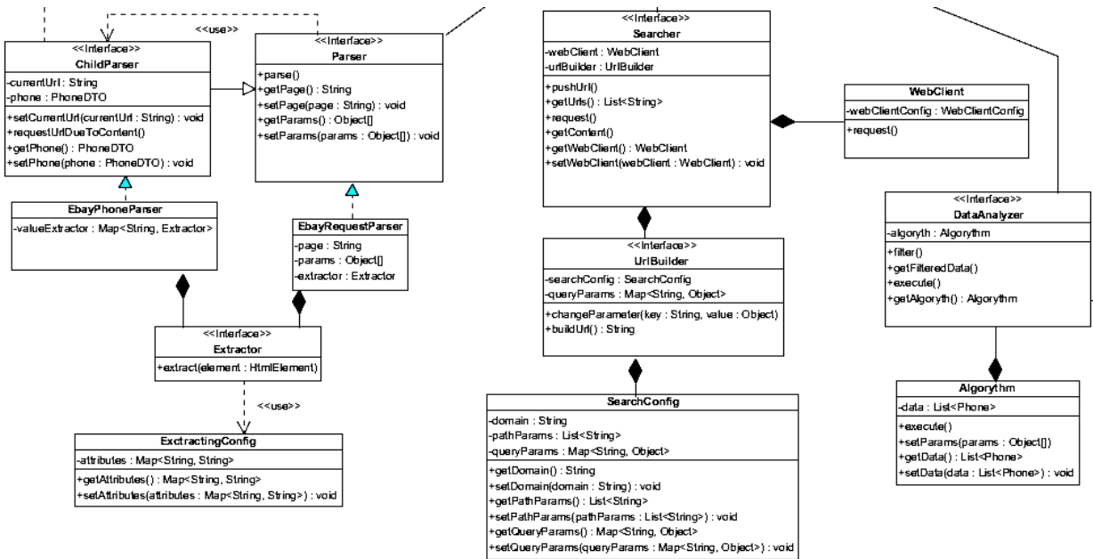
Fig. 5. Domain layer
