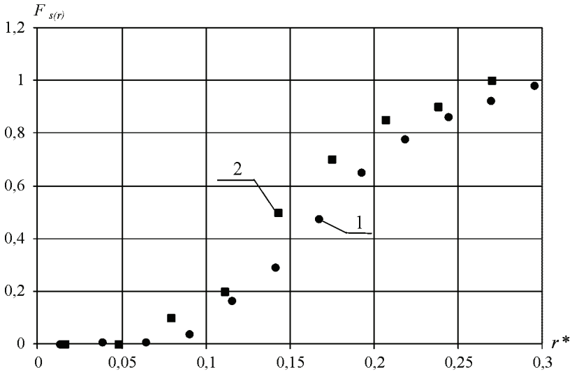
Рисунок 9 – Эмпирические функции распределение точек поражения заземленной плоскости: 1 – эксперимент №3; 2 – эксперимент №4
