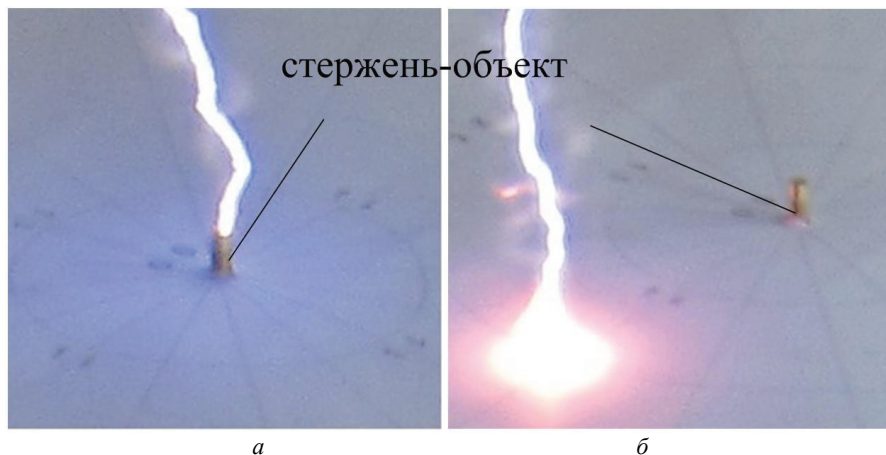
Рисунок 8 – фрагмент пробоя РП с поражением стержня-объекта и мишени: а – поражение стержня-объекта; б – поражение мишени
