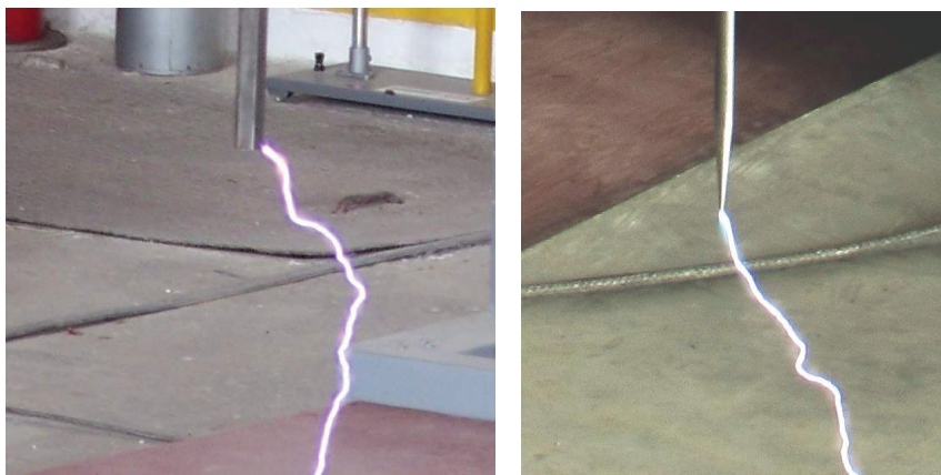
Рисунок 5 – Формирование разряда при различной форме электрода: а – шестигранник с плоским торцом; б – цилиндрический с заостренным торцом
