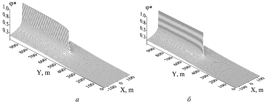
Рисунок 3 – Рассчитанные распределения потенциала. a - модель «заряд, равномерно распределенный по нити»; б - модель «заряженный эллипсоид»
