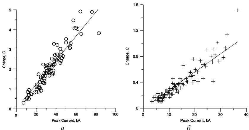
Рисунок 1 – Заряд лидерного канала молнии, нейтрализованный в первые 100 мкс ( a ) и 50 мкс ( б ) возвратного удара [2 - 4]
