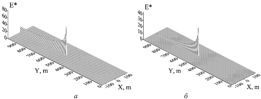
Рисунок 4 – Рассчитанные распределения напряженности ЭП E = |E|/E_{\text{вaz}} : а - модель «заряженный эллипсоид»; б - модель «эллипсоид во внешнем однородном ЭП»
