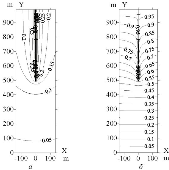
Рисунок 2 – Рассчитанные распределения линий равного потенциала \varphi^* = \varphi/U_L : а - модель «заряженный эллипсоид»; б - модель «эллипсоид во внешнем однородном ЭП»
