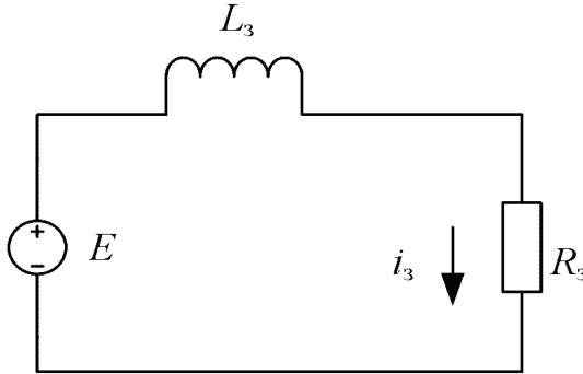
Рисунок 1 – Упрощенная электрическая схема трансформатора с индуктивным накоплением
