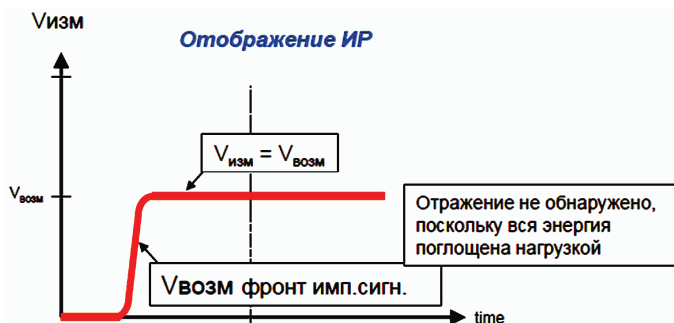
Рисунок 5 – Форма отраженного импульса при согласованной нагрузке ( Z_n = Z_0 )
