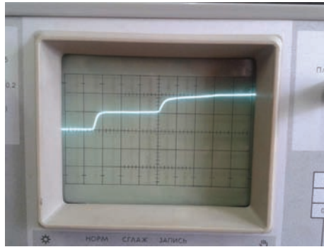
Рисунок 11 – Форма отраженного импульса при подключении входной цепи оптического передатчика
