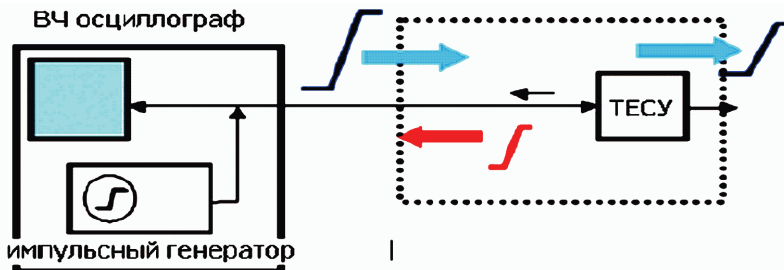
Рисунок 2 – Структурная схема измерения на принципе ИР
