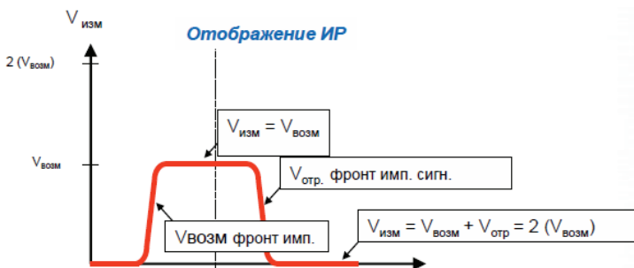
Рисунок 4 – Форма отраженного импульса при коротком замыкании ( Z_n = 0 )
