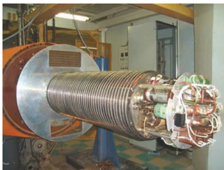
Рисунок 1 – ЭСУ «СОКОЛЬ» без кондуктора и сосуда высокого давления
