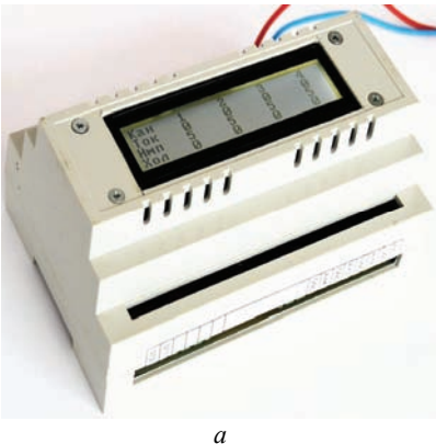
Рисунок 7 – Зовнішній вигляд пристрою системи моніторингу поточного стану ГС: a – система моніторингу із функцією струмового захисту; б – результати вимірювання розрядного струму і кількості зарахованих імпульсів в кожному з чотирьох каналів розряду при випробуваннях пристрою
