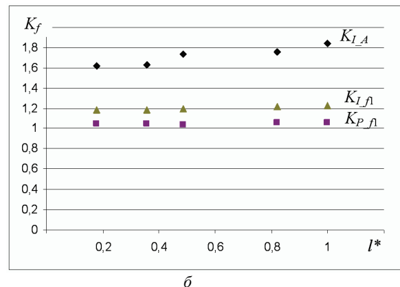
Рисунок 5 – Залежності коефіцієнтів форми імпульсів напруги K_U (а) та форми імпульсів струму K_I й потужності K_P (б) від довжини міжелектродного проміжку l^*
