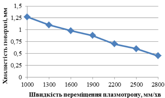
Рис. 2 – Залежність хвилястості поверхні розрізу від швидкості переміщення плазмоторону
