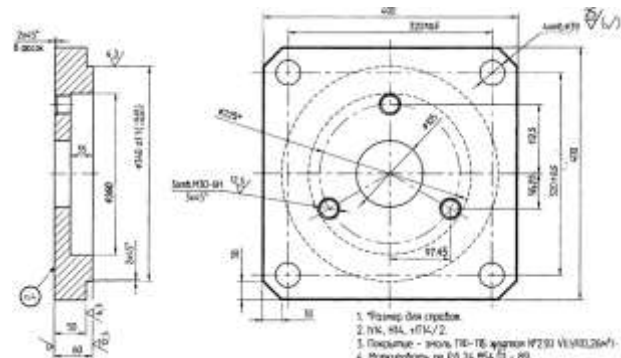
Рис. 1 – Деталь «Крышка»
