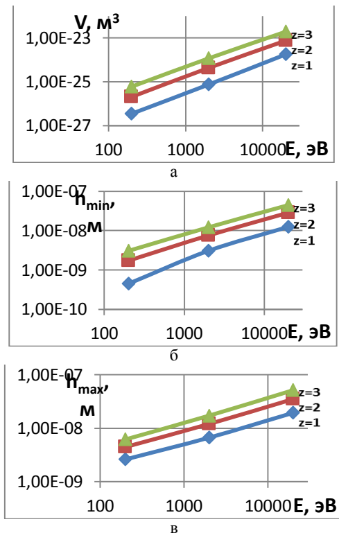
Рис. 8 – Зависимости объёма НК (а), минимальной (б) и максимальной (в) глубины залегания НК при действии ионов никеля ( \text{Ni}^+ ) с различным зарядом ( z = 1, z = 2, z = 3 ) для СТМ кортинита
