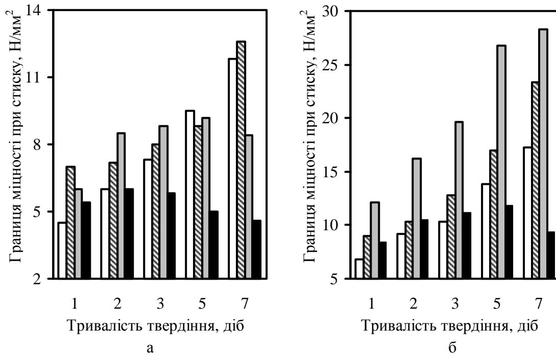
Рис. 2 – Механічна міцність перикалазового бетону на ранніх стадіях твердіння: а – бетон з матрицею № 1, б – бетон з матрицею № 2. Тривалість подрібнення перикалазу і матриці: □ – 5 хв., ▨ – 10 хв., ▣ – 15 хв., ■ – 20 хв.
