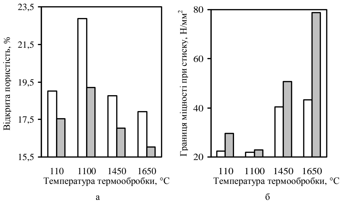
Рис. 3 – Показники властивостей перикалазового бетону після термічної обробки: твердіння: а – відкрита пористість, б – границя міцності при стиску. (□ – бетон з матрицею № 1, ▣ – бетон з матрицею № 2).
