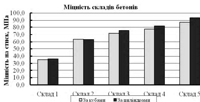
Рисунок 1 – Міцність складів бетонів визначена на зразках-кубах та циліндрах.
