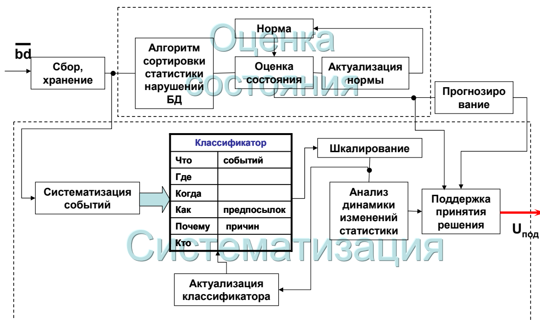
Рис. 3 Структура метода статистической закономерности в управлении безопасностью движения
