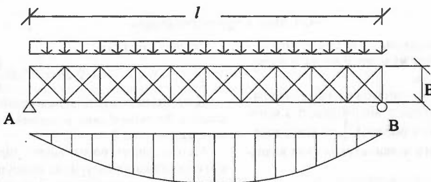
Рис. 3. Епюра балочних моментів
