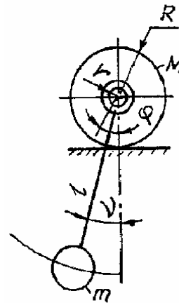
Рис. 3. Расчетная схема
